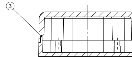
SCHNITT A-A
